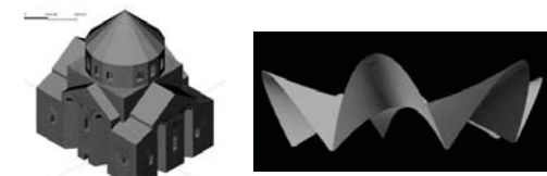
図14 Hripsime 補強検討 図15: Xochimilco 構造モデル
