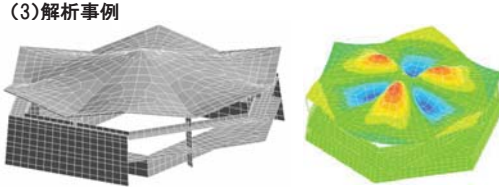
図8: RCシェル構造設計への技術協力(豊島美術館)*H23竣工
