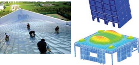
図1: 建造物の安全性評価へ取り組み(左:測定 右:解析)
