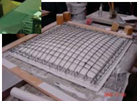
図6: RC自由曲面の試験体
