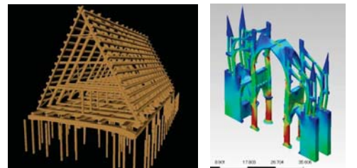
図13: 合掌造の再現モデルCG ゴシック聖堂の解析
